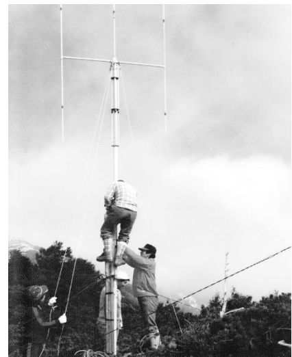
S 55 年大町報話局線路宅内課時代に 夏山無線取り付け工事の写真
